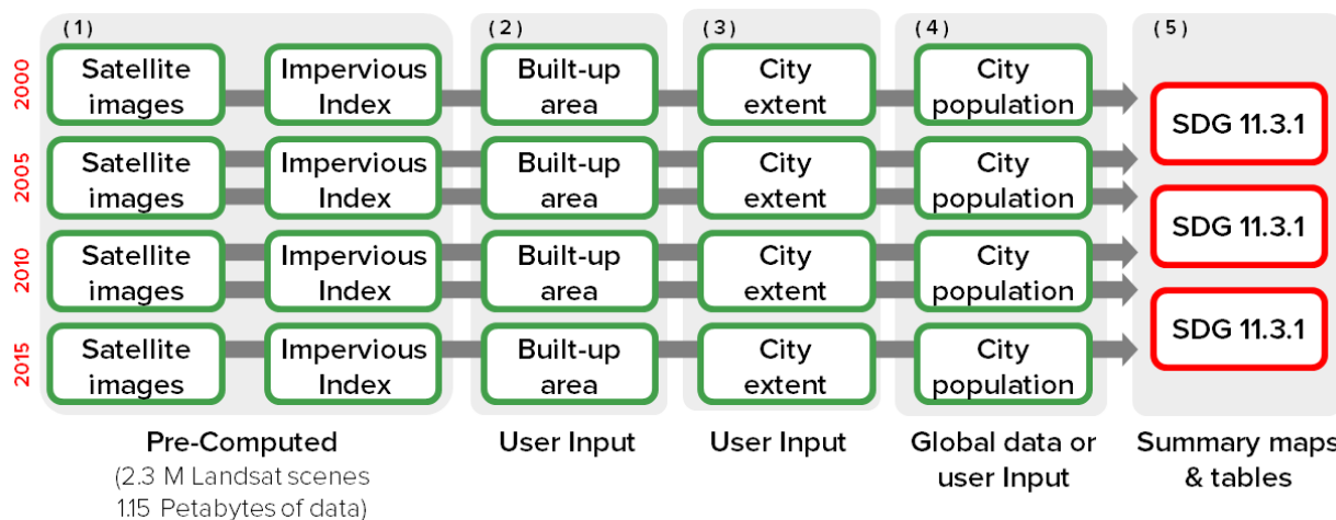
Figura 2: Fluxo de trabalho do Trends.Earth para calcular o ODS 11.3.1. Os índices globais de superfícies impermeáveis de 30 m foram pré-calculados e estão disponíveis para os utilizadores explorarem no Trends.Earth Urban Mapper , onde o utilizador define a extensão construída simplesmente atribuindo uma série de limites.
