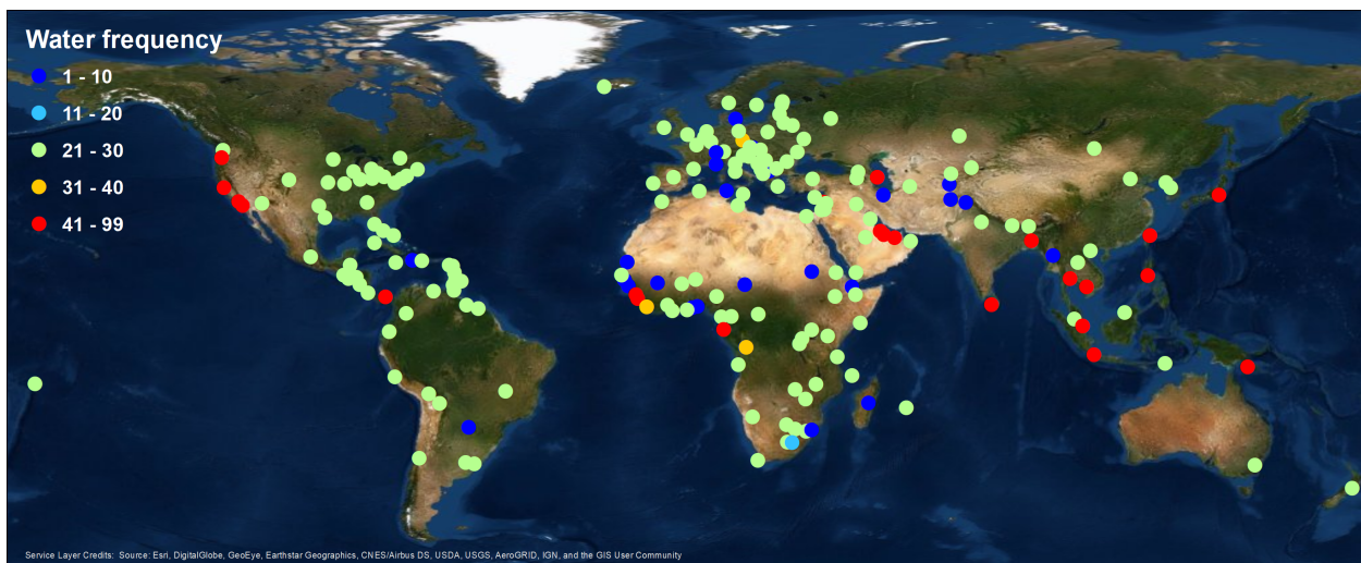
Figura 8: Distribuição espacial dos parâmetros de limiar selecionados para a amostra de 224 cidades testadas. Parte superior: Indicador de área de superfície impermeável, meio: indicador de luzes noturnas e inferior: indicador de frequência de água.
